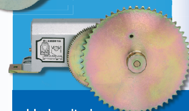
Hydraulische Schiebetür-Schliesser mit Umlenkrollen in entsprechenden Grössen
